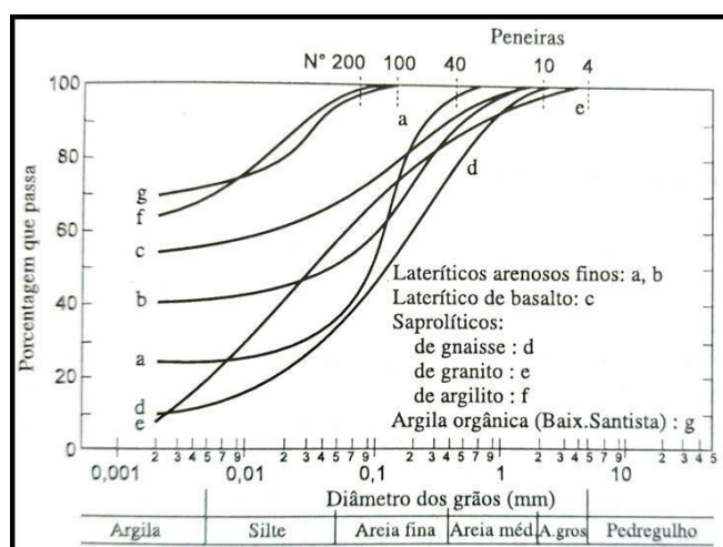
Figura 01: Curvas granulométricas
